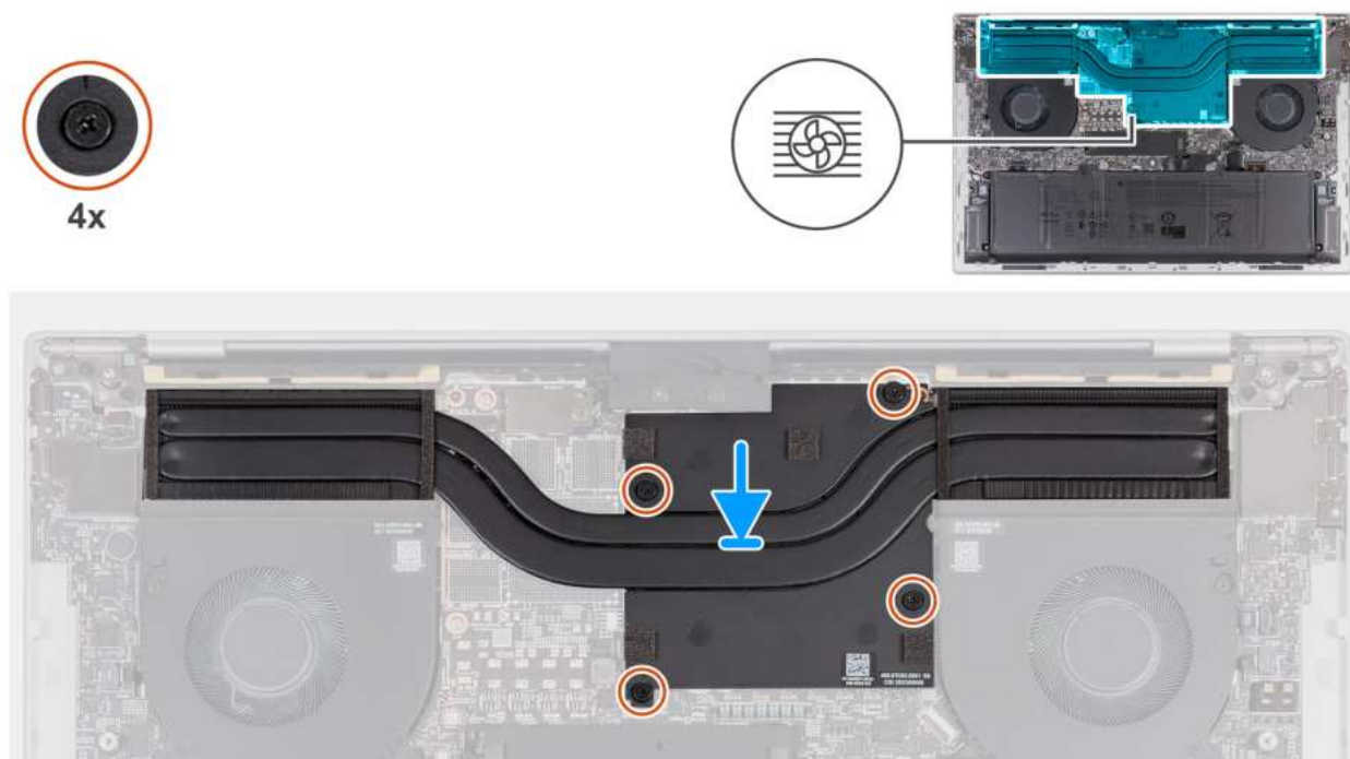
Rysunek 32. Instalowanie radiatora — konfiguracja ze zintegrowaną kartą graficzną
