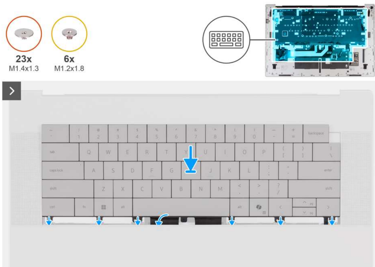
Rysunek 59. Instalowanie klawiatury
