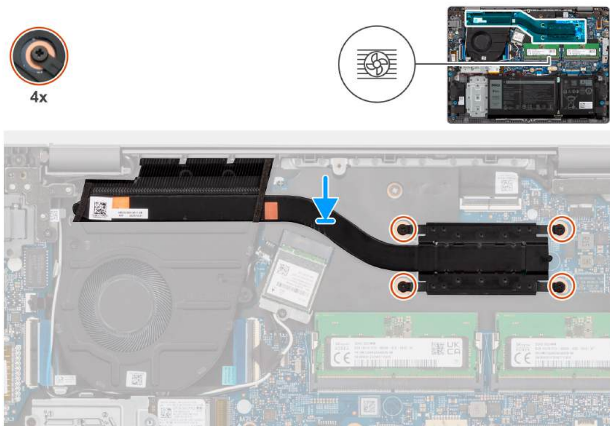
Rysunek 27. Instalowanie radiatora
