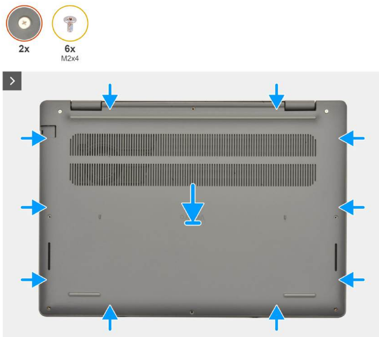
Rysunek 12. Instalowanie pokrywy dolnej
