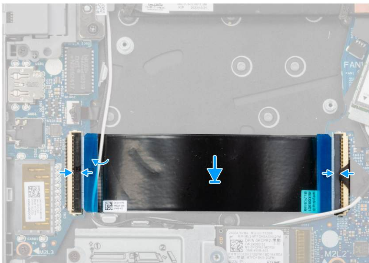
Rysunek 35. Instalowanie kabla płyty we/wy
