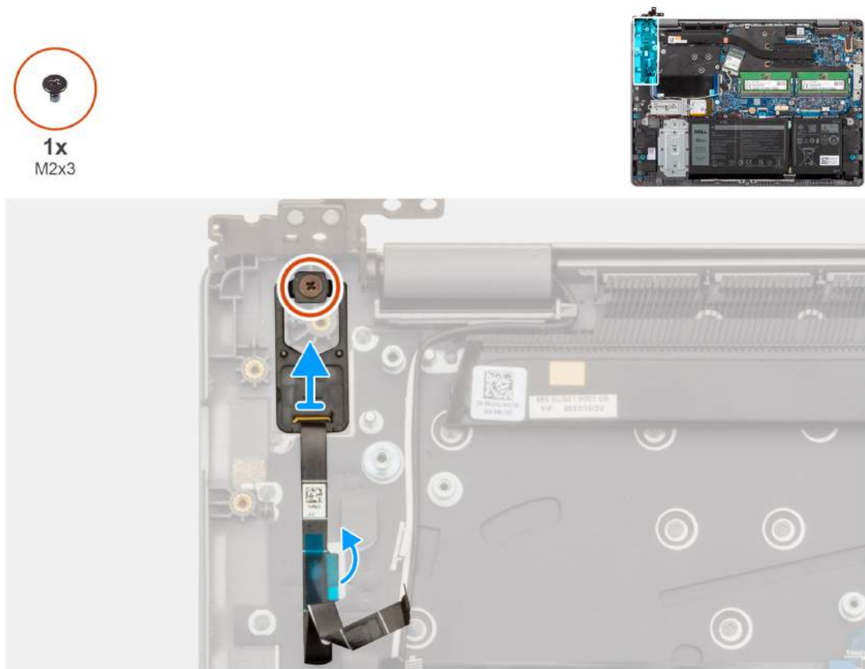
Rysunek 40. Wymontowywanie przycisku zasilania z opcjonalnym czytnikiem linii papilarnych
