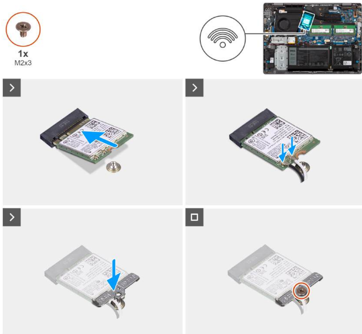
Rysunek 19. Instalowanie karty sieci bezprzewodowej
