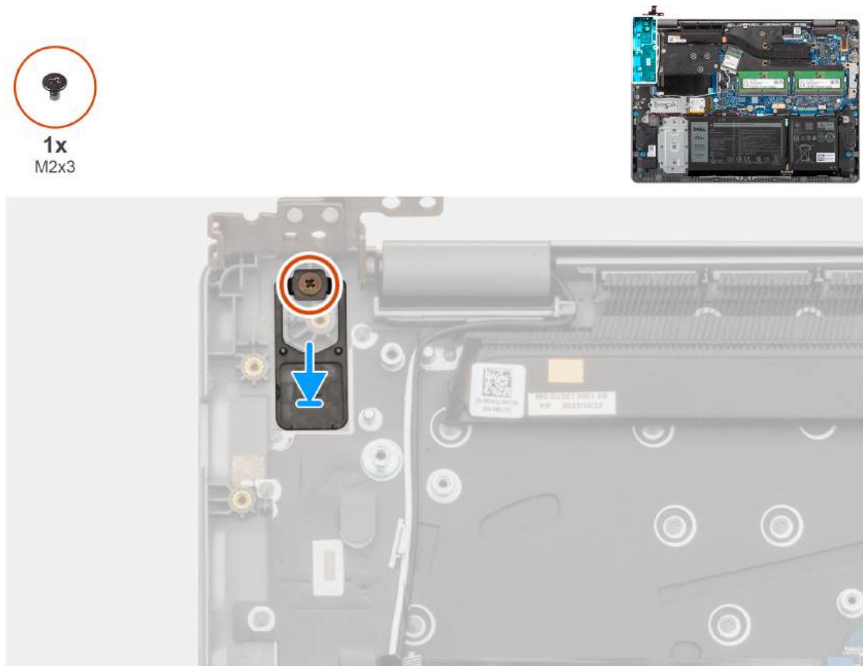
Rysunek 39. Instalowanie przycisku zasilania
