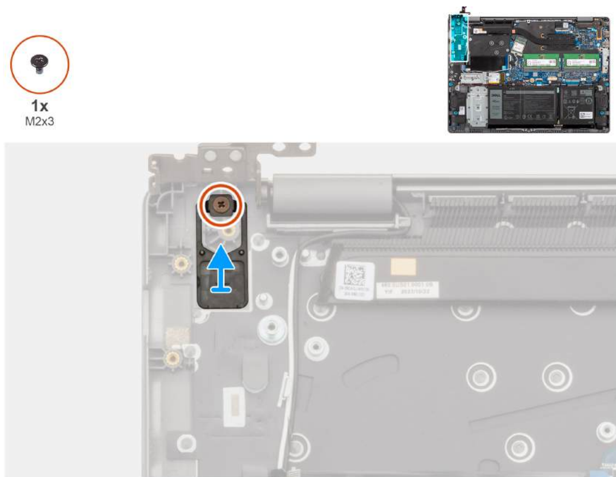
Rysunek 38. Wymontowywanie przycisku zasilania
