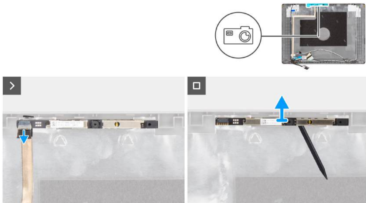
Rysunek 64. Wymontowywanie kamery
