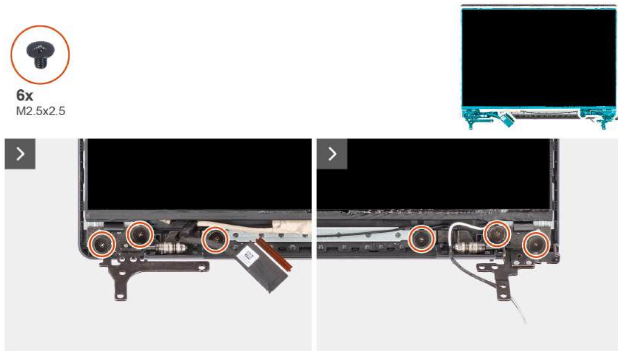
Rysunek 53. Wymontowywanie wyświetlacza
