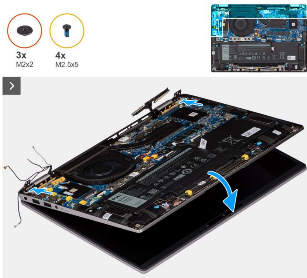
Rysunek 50. Instalowanie zestawu wyświetlacza
