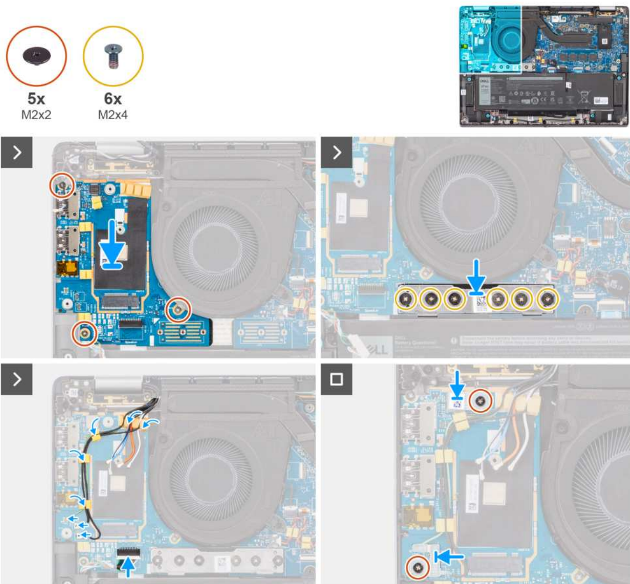
Rysunek 72. Instalowanie karty towarzyszącej we/wy
