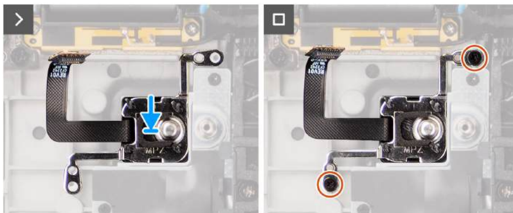
Rysunek 63. Instalowanie przycisku zasilania z opcjonalnym czytnikiem linii papilarnych
