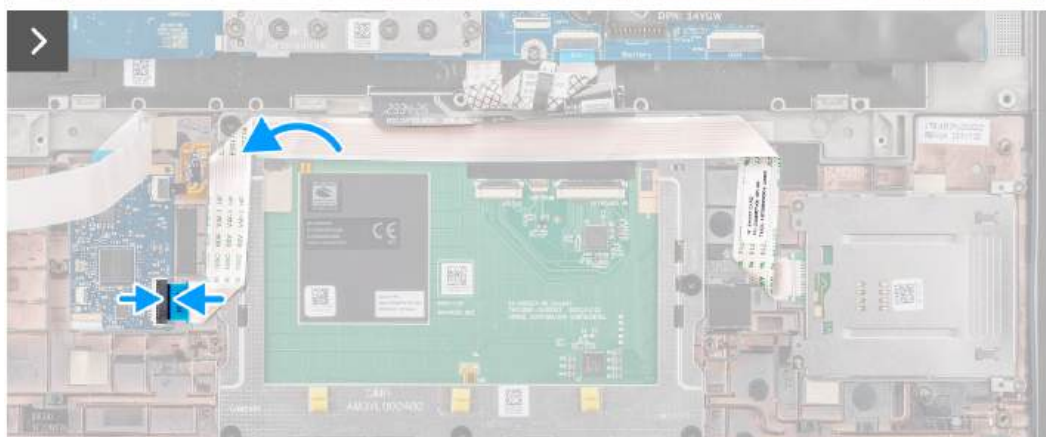
Rysunek 44. Instalowanie czytnika kart smart
