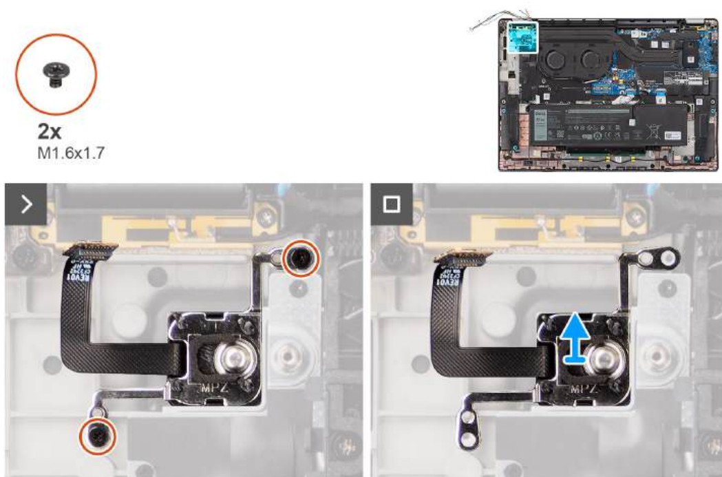
Rysunek 62. Wymontowywanie przycisku zasilania z opcjonalnym czytnikiem linii papilarnych
