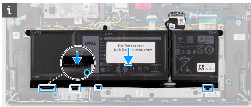
Rysunek 31. Instalowanie baterii — wkładanie wypustek do zaczepów
