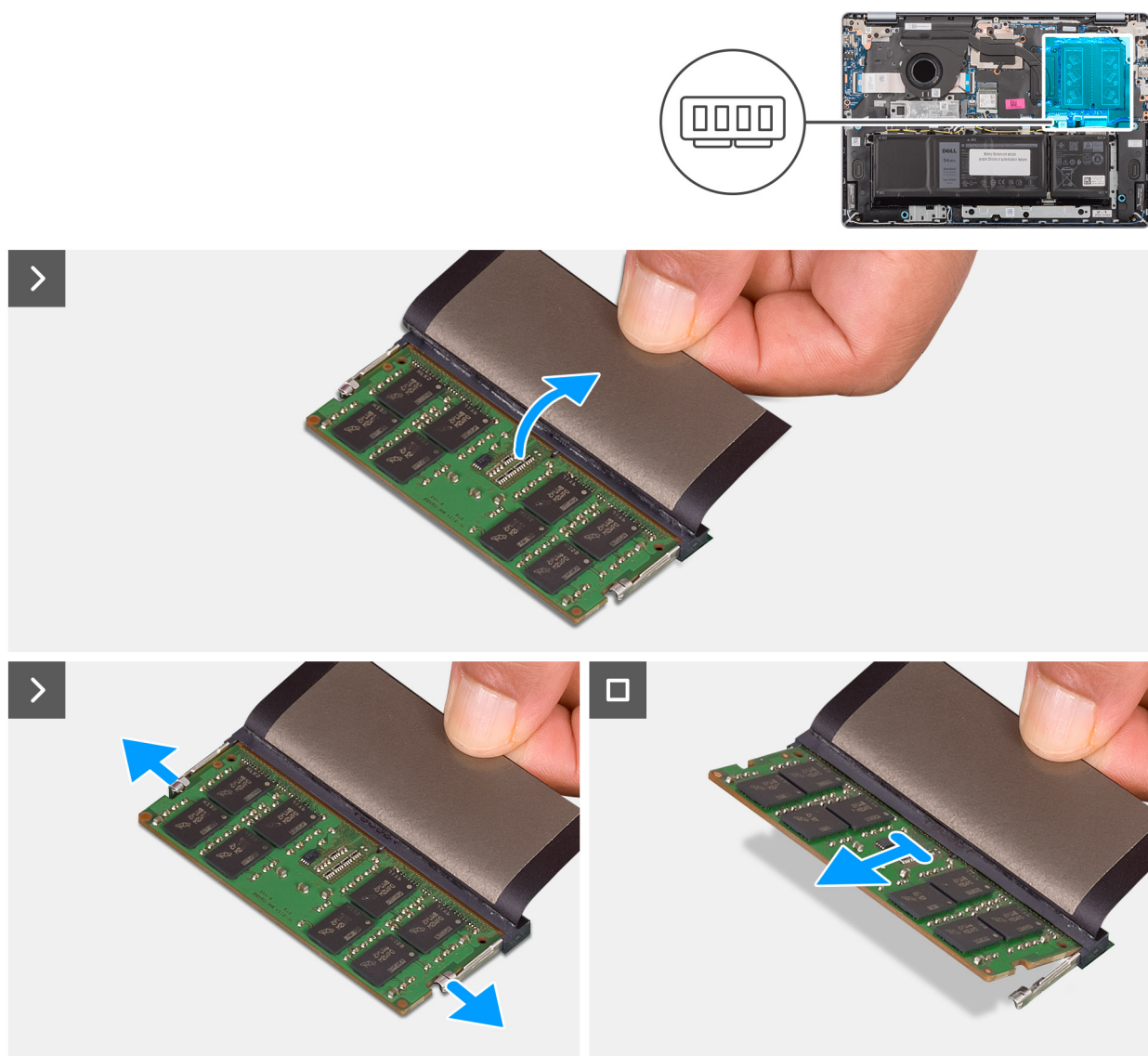
Rysunek 13. Wymontowywanie modułu pamięci
