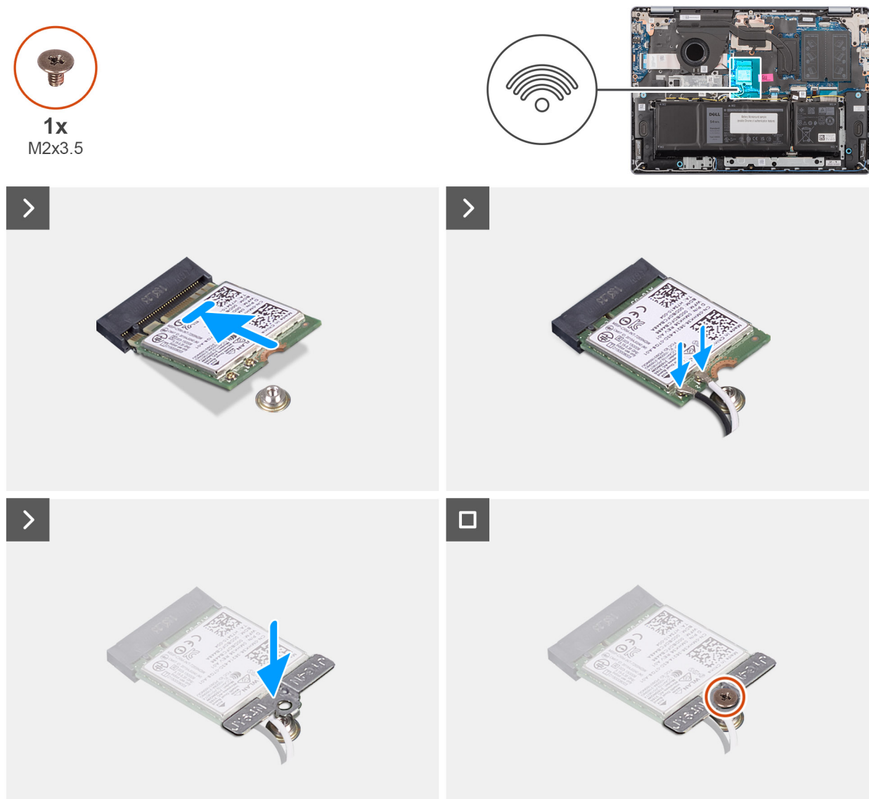
Rysunek 18. Instalowanie karty sieci bezprzewodowej
