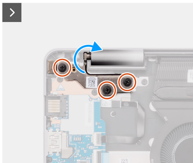
Rysunek 42. Wykręcanie śrub zawiasów i odłączanie kabla wyświetlacza
