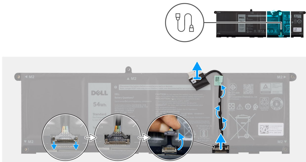
Rysunek 28. Odłączanie kabla baterii
