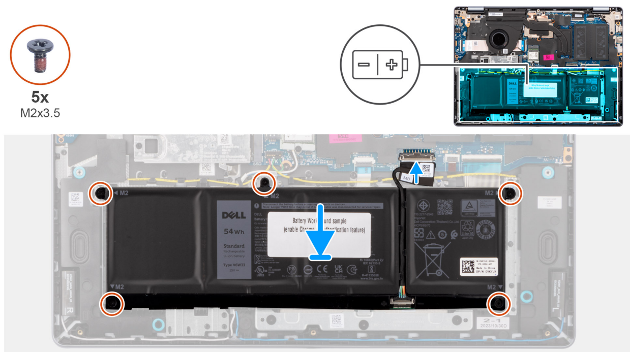
Rysunek 30. Instalowanie baterii
