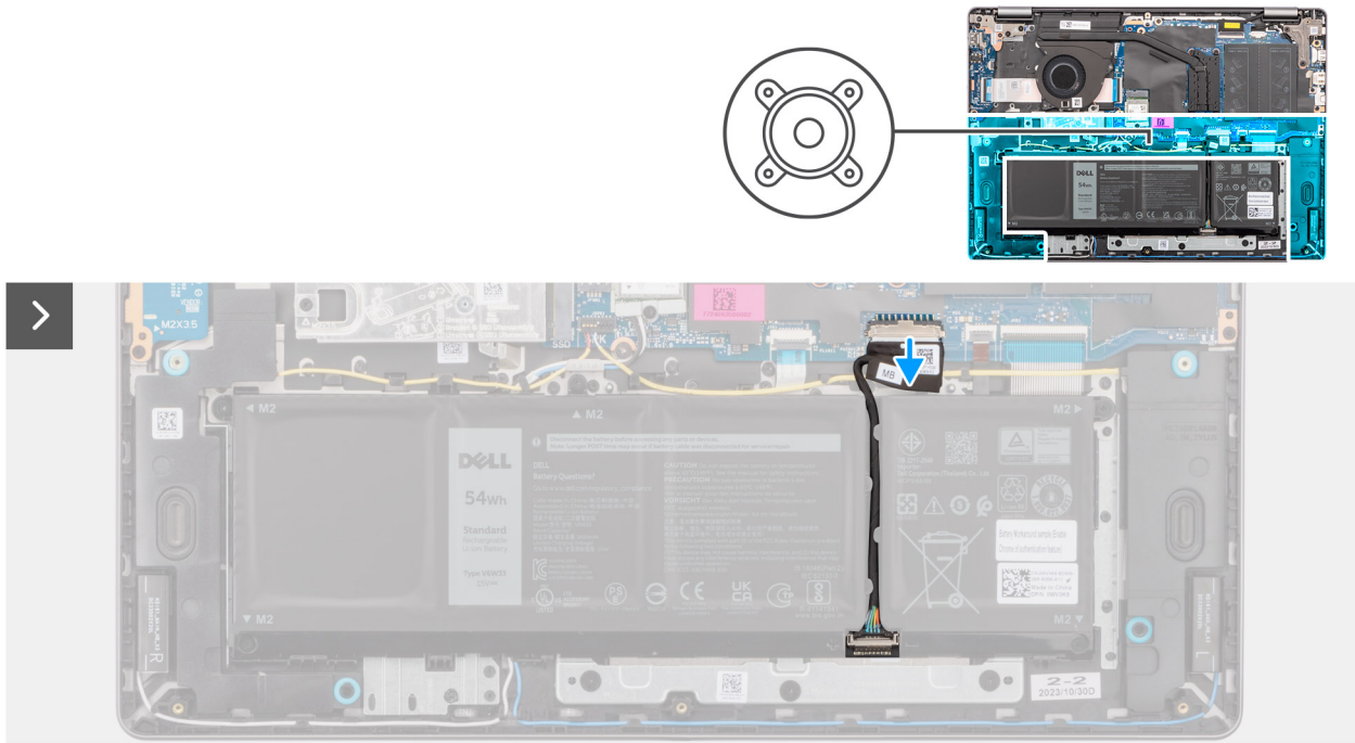
Rysunek 19. Odłączanie kabla baterii
