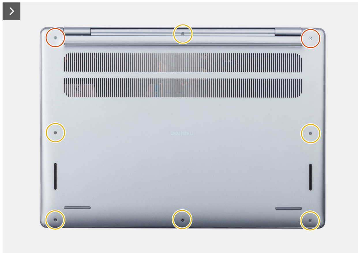
Rysunek 9. Wymontowywanie pokrywy dolnej
